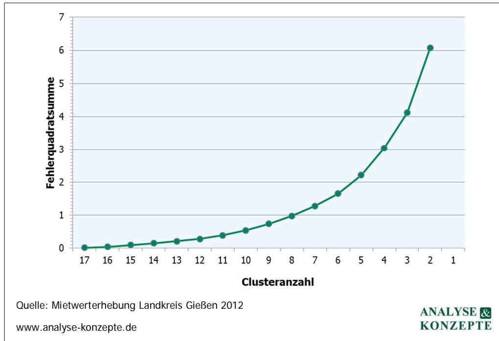
Abb. A21 Entwicklung der Fehlerquadratsumme der Clusterlösungen für die Wohnungsmarkttypen im Landkreis Gießen
