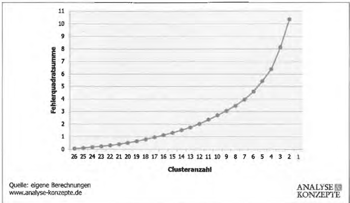
Abb. A21 Entwicklung der Fehlerquadratsumme der Clusterlösungen für die Wohnungsmarkttypen im Schwalm-Eder-Kreis
